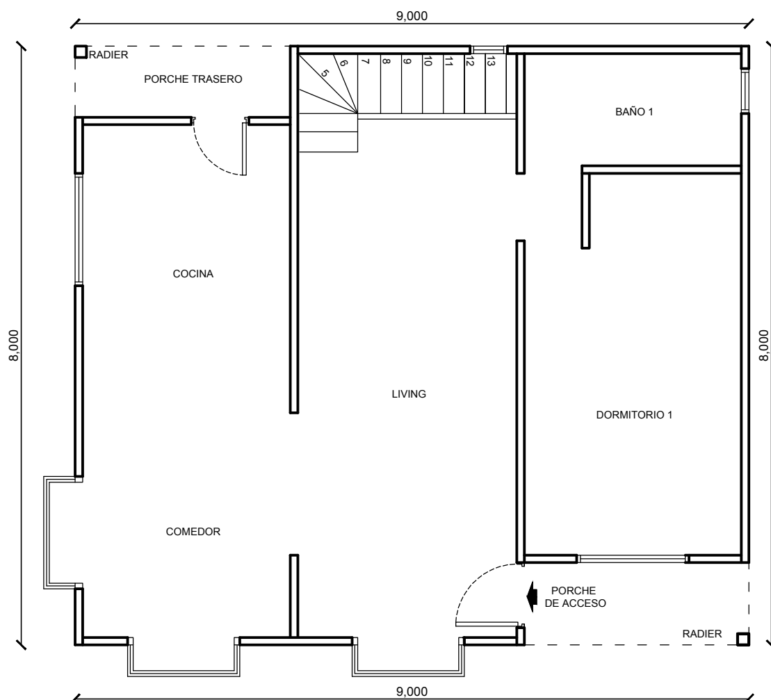
PLANO DE DISTRIBUCIÓN PRIMER NIVEL CASA MODELO ANTONIA 118m 2
