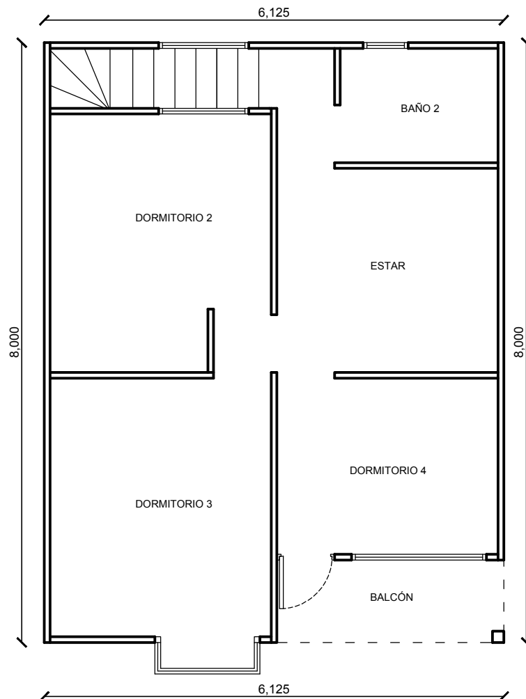
PLANO DE DISTRIBUCIÓN SEGUNDO NIVEL CASA MODELO ANTONIA 118m 2
